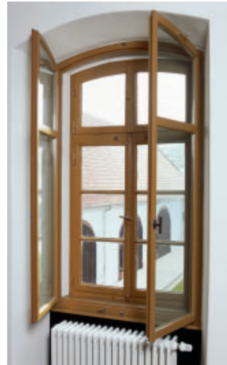
9 Instandgesetztes und zum Kastenfenster umgebautes historisches Fenster.
